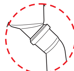
45° Senkrechtabgang durch Umdrehen des Bogens
